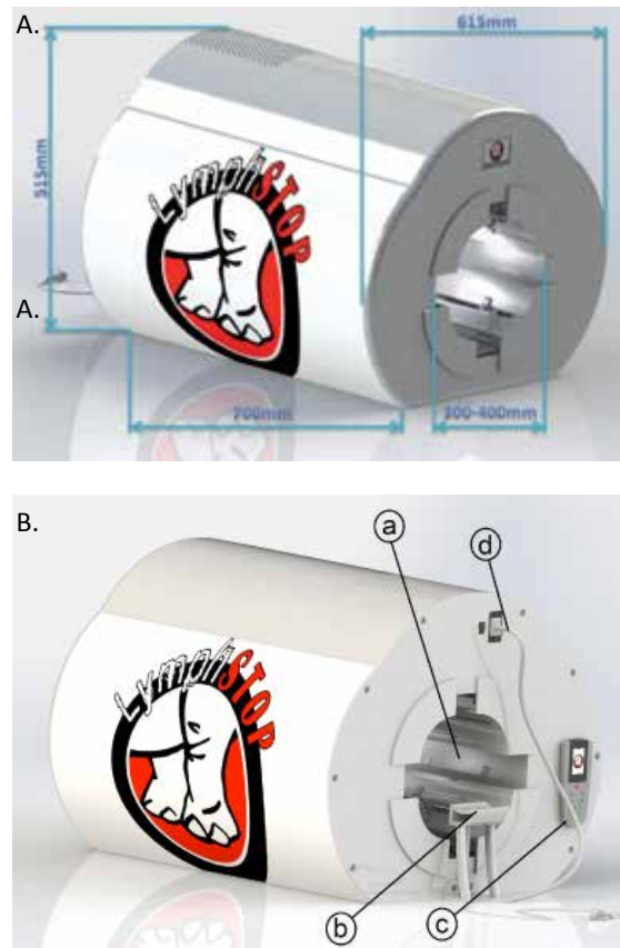
Rysunek 1. Studium projektowe biomechatronicznego aparatu wspomagającego drenaż limfatyczny kończyn dolnych i górnych „LymphSTOP”: A) widok z przodu z wymiarami gabarytowymi, B) widok z tyłu: a – 4-częściowy kanał wewnętrzny, b – podpórka pod kończynę dolną, c – pilot bezprzewodowy, d – kabel zasilający
