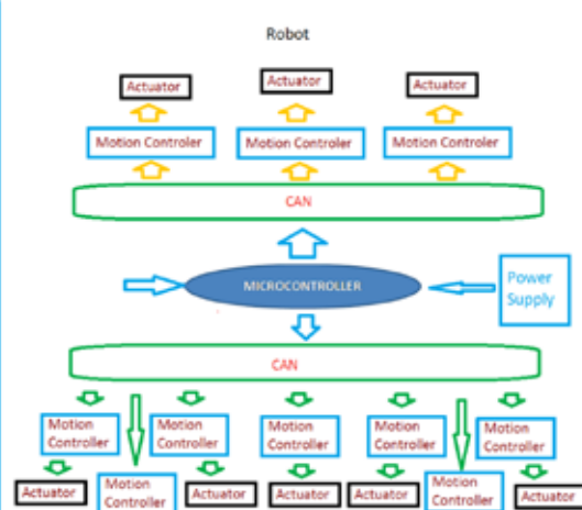
Rysunek 5. Schemat blokowy systemu Robin Heart Tele
